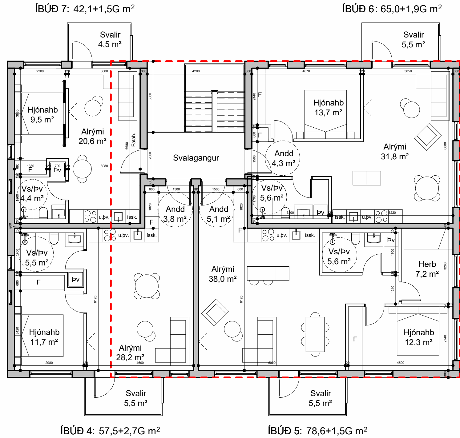
2.hæð mkv: 1 : 100
